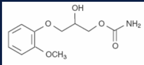
methocarbamol
